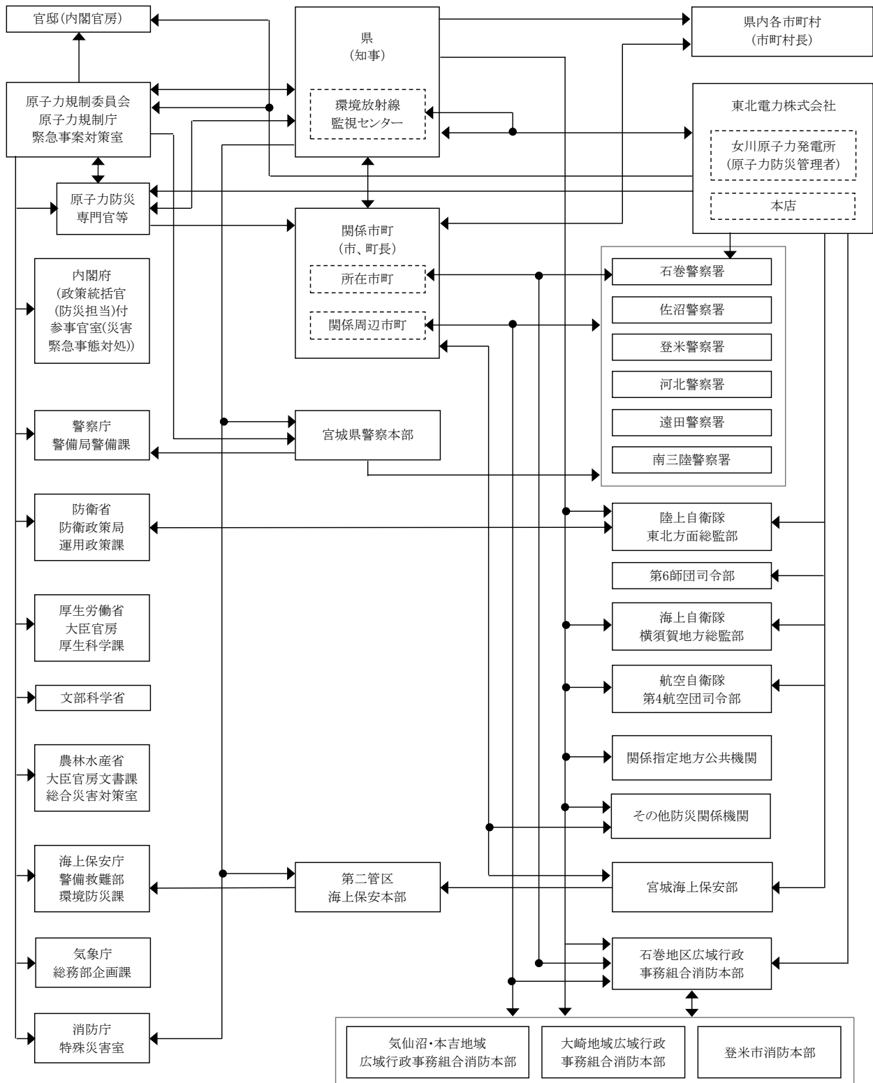
図 3 - 2 - 1 緊急時通報連絡系統図
