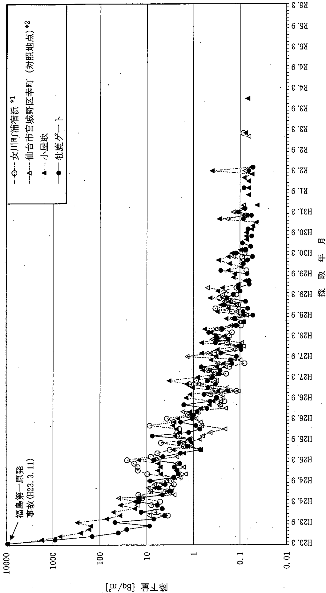
図-2-1-19 福島第一原発事故後のCs-134の月間降水量の推移
