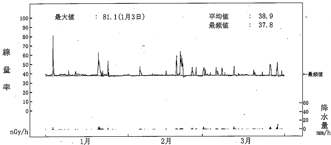
図-2-9 NaI(Tl)検出器による空間ガンマ線量率監視結果(寺間局) (注) 3月18日~19日の欠測は、機器更新によるものである。
