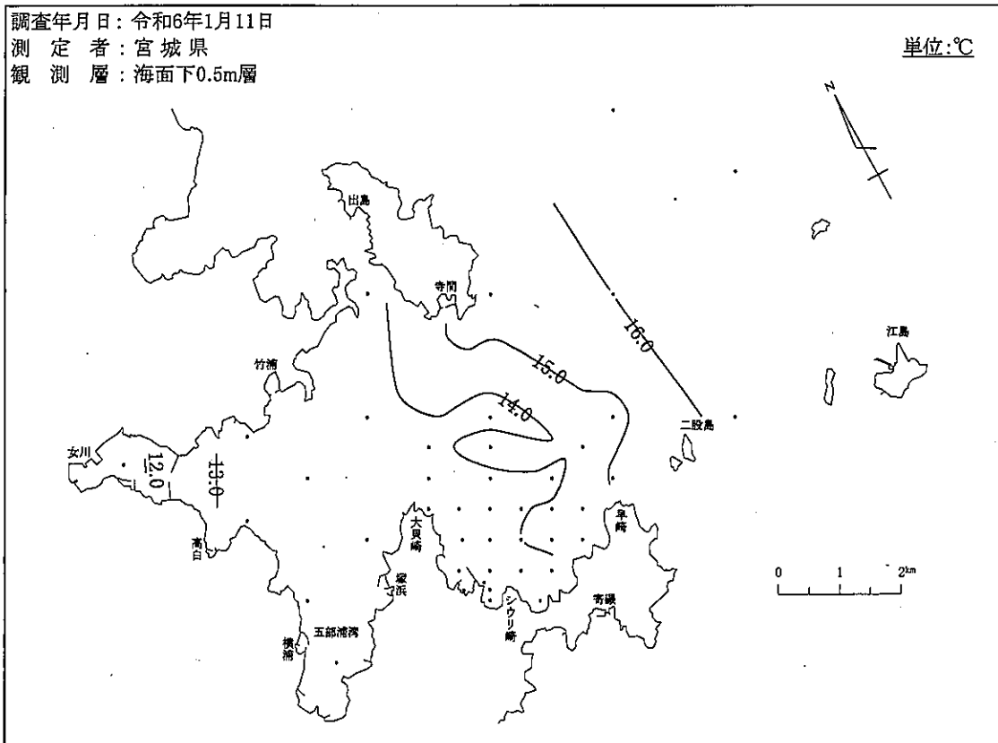
図-2-(2) 等温線
