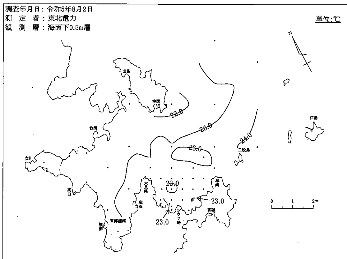
図-4-(2) 等温線
