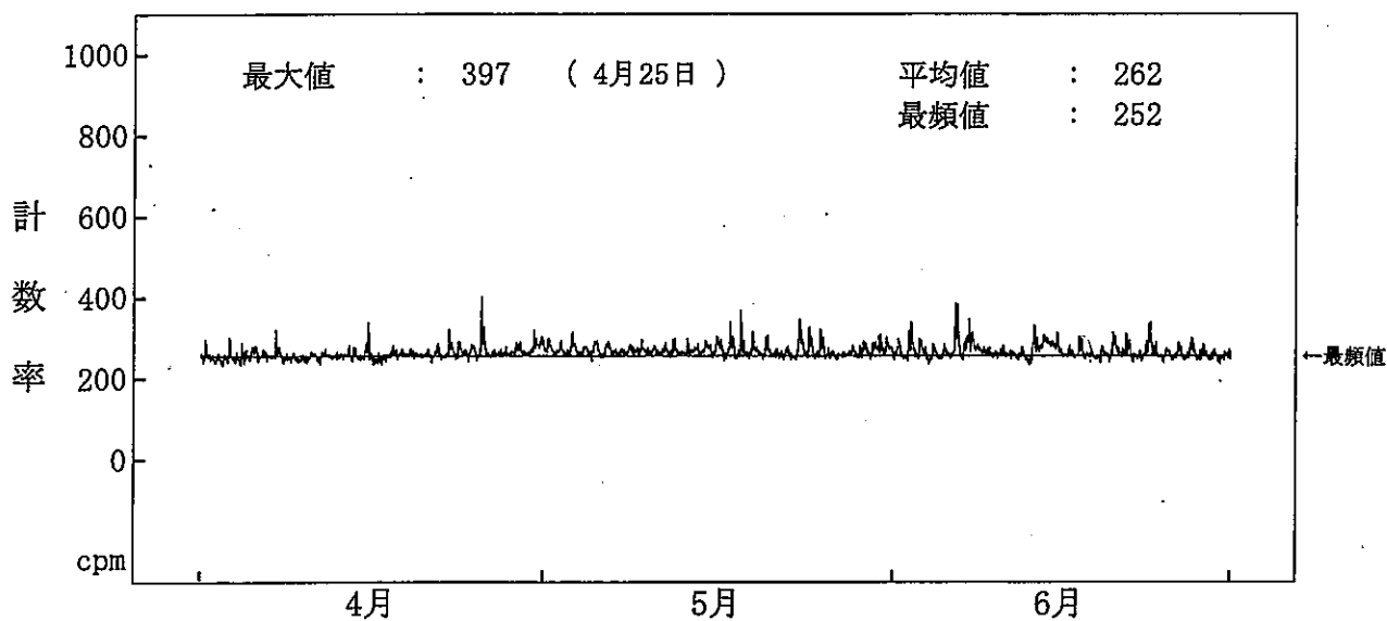
図-2-13 海水(放水)中の全ガンマ線計数率監視結果(1号機放水口モニター(B)) (注) 6月1日の欠測は、定期点検によるものである。
