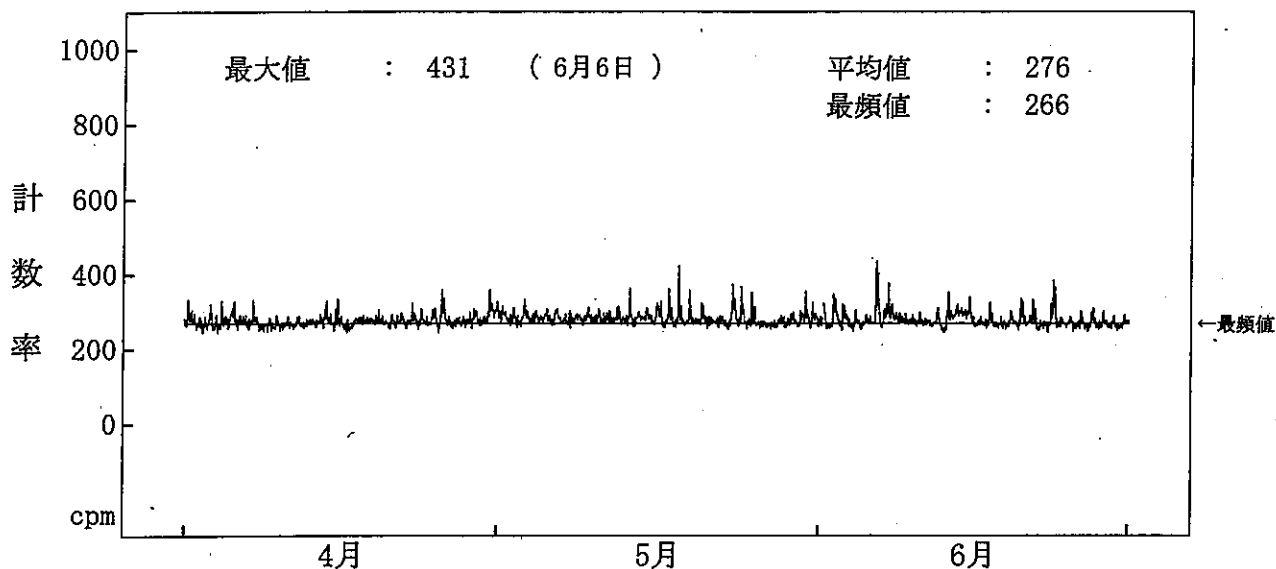
図-2-12 海水(放水)中の全ガンマ線計数率監視結果(1号機放水口モニター(A)) (注) 6月1日の欠測は、定期点検によるものである。
