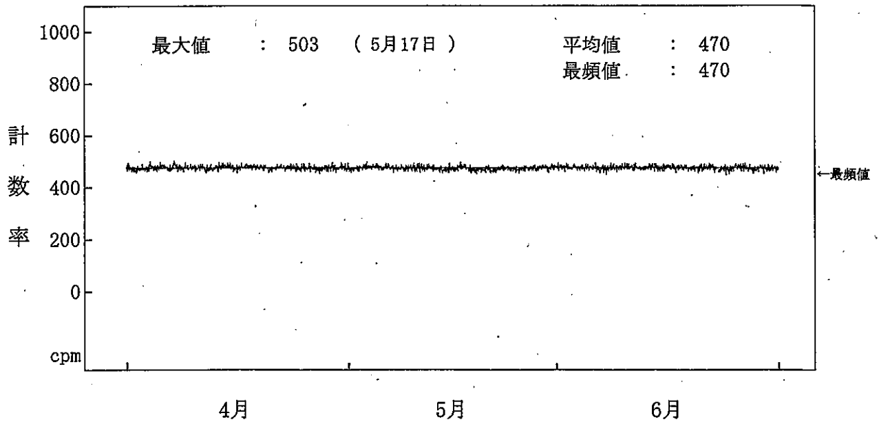
図-2-11 海水(放水)中の全ガンマ線計数率監視結果(3号機放水口モニター) (注) 4月20日、5月18日、6月22日の欠測は、定期点検によるものである。
