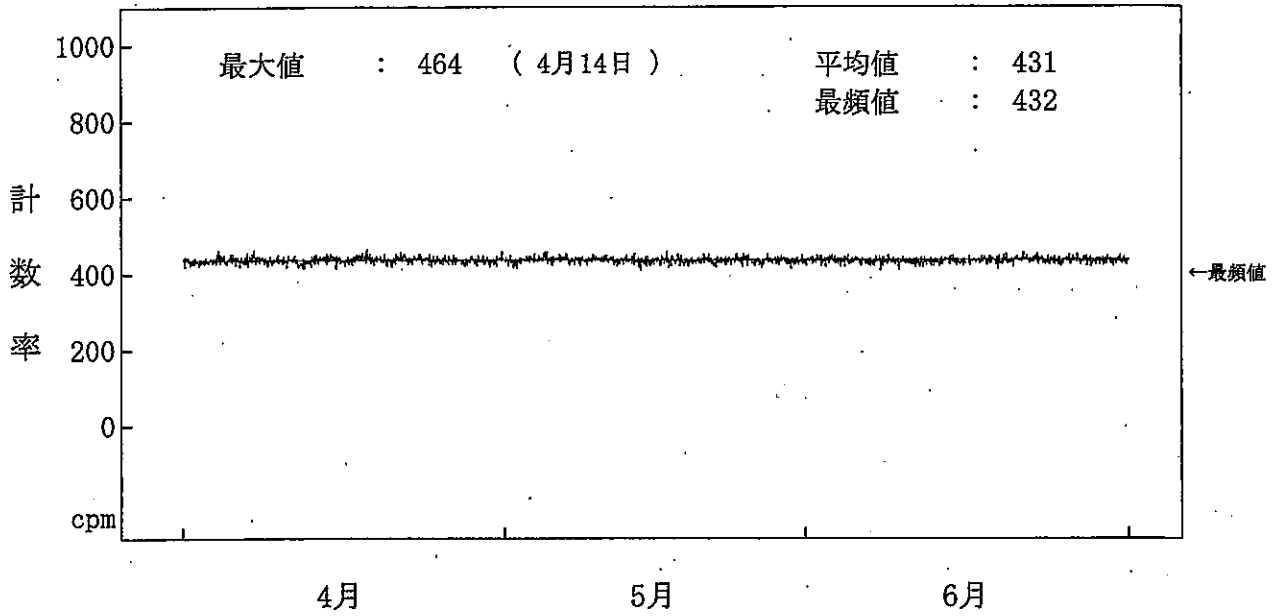
図-2-10 海水(放水)中の全ガンマ線計数率監視結果(2号機放水口モニター) (注) 4月27日、5月25日、6月15日の欠測は、定期点検によるものである。
