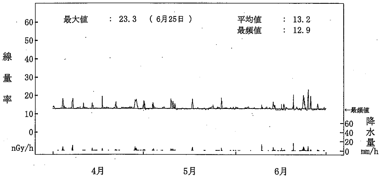
図-2-5 空間ガンマ線線量率監視結果 (寺間局) (注) 下方を鉛で遮へいたNaI (T1) 検出器により測定した。
