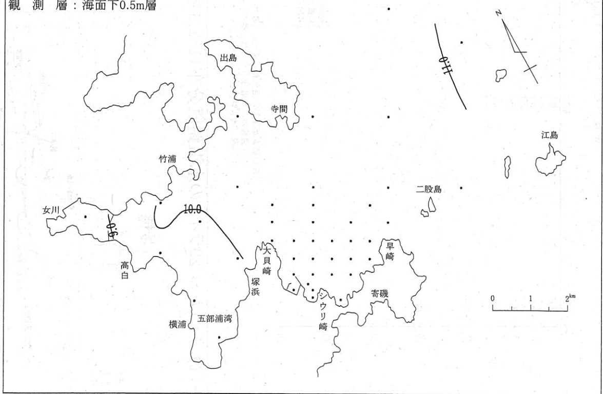
図-2-(2) 等温線
