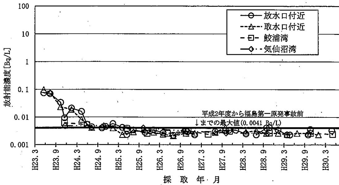
図-2-21 海水のCs-137濃度の推移
