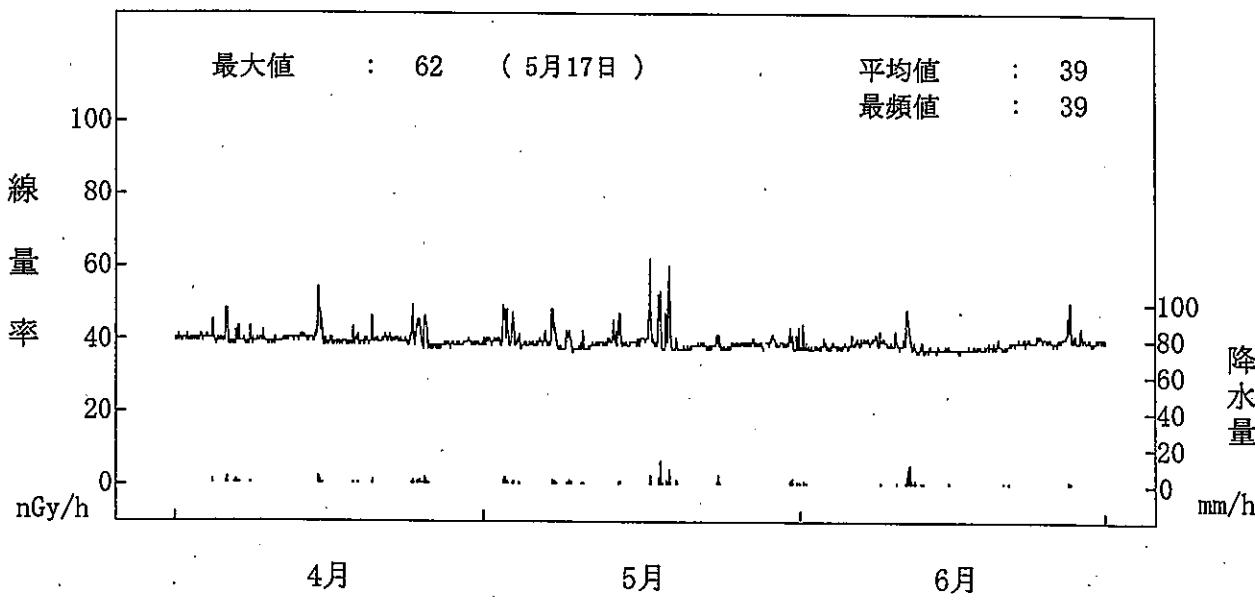
空間ガンマ線線量率監視結果(MP-2)
