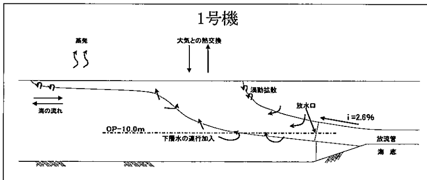
図-3-(2) 水中放流方式における温排水の拡散概念
