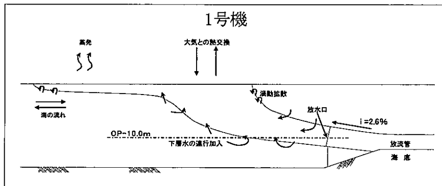
図-5-(2) 水中放流方式における温排水の拡散概念
