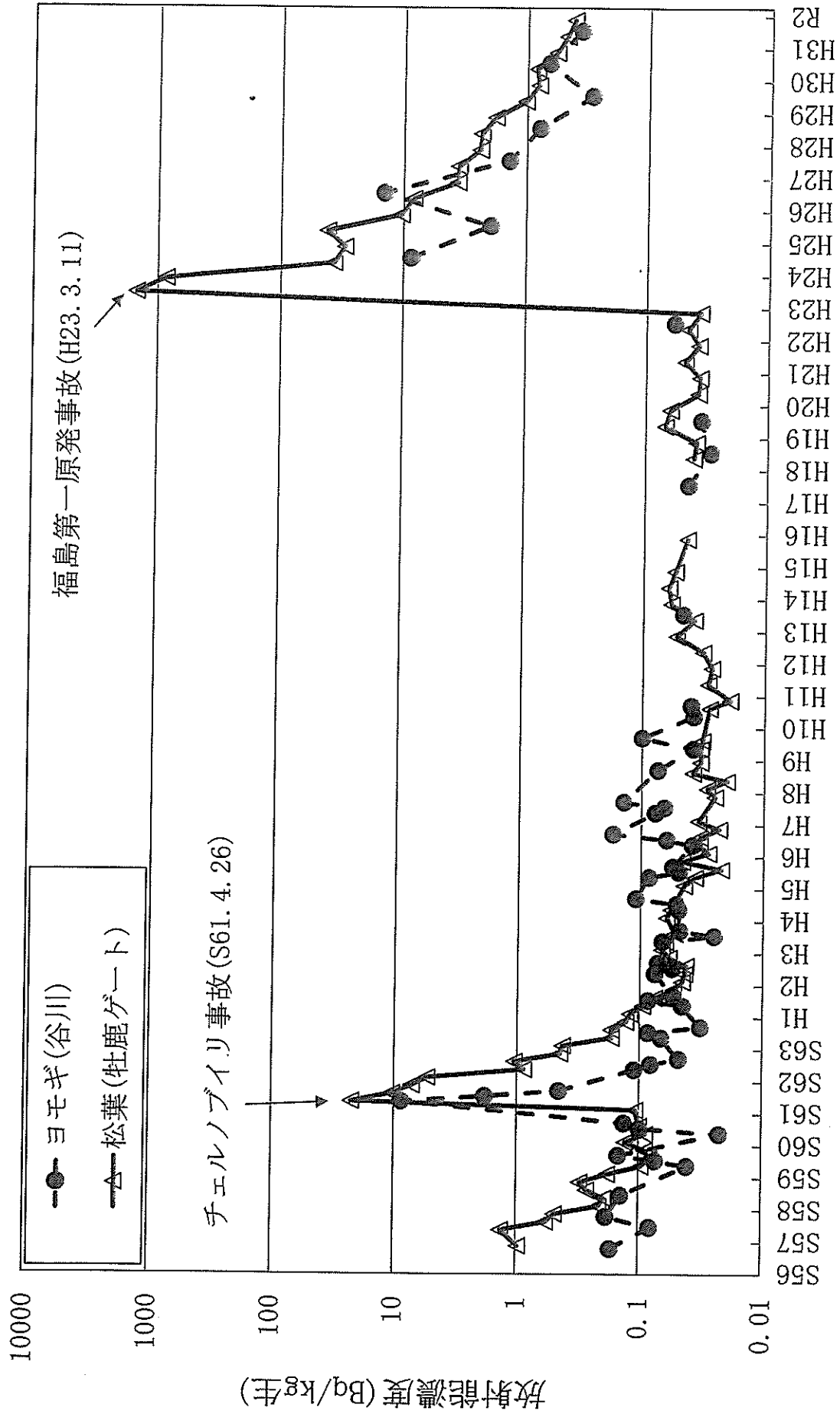
図-3 陸上試料中のCs-137濃度の推移
