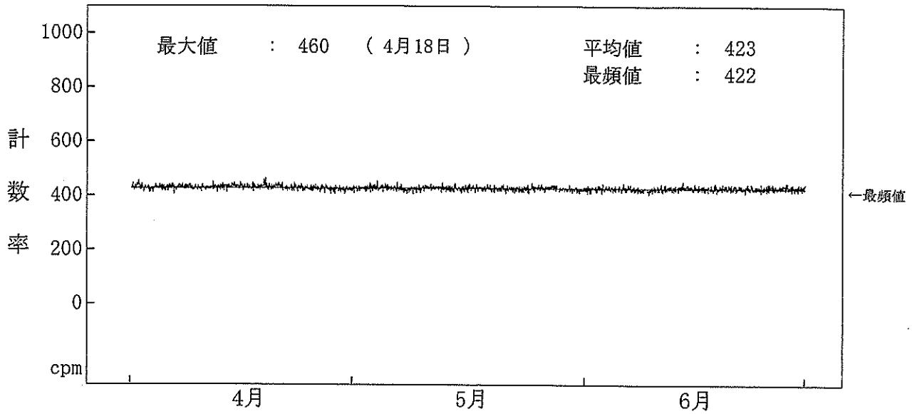
図-2-14 海水(放水)中の全ガンマ線計数率監視結果(2号機放水口モニター) (注) 4月21日、5月28日及び6月9日の欠測は、定期点検によるものである。
