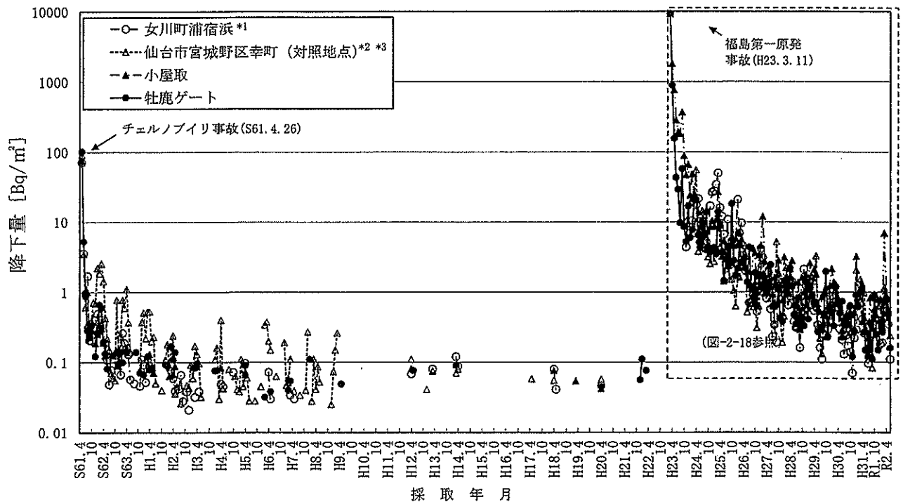
図-2-16 Cs-137の月間降下量の推移
