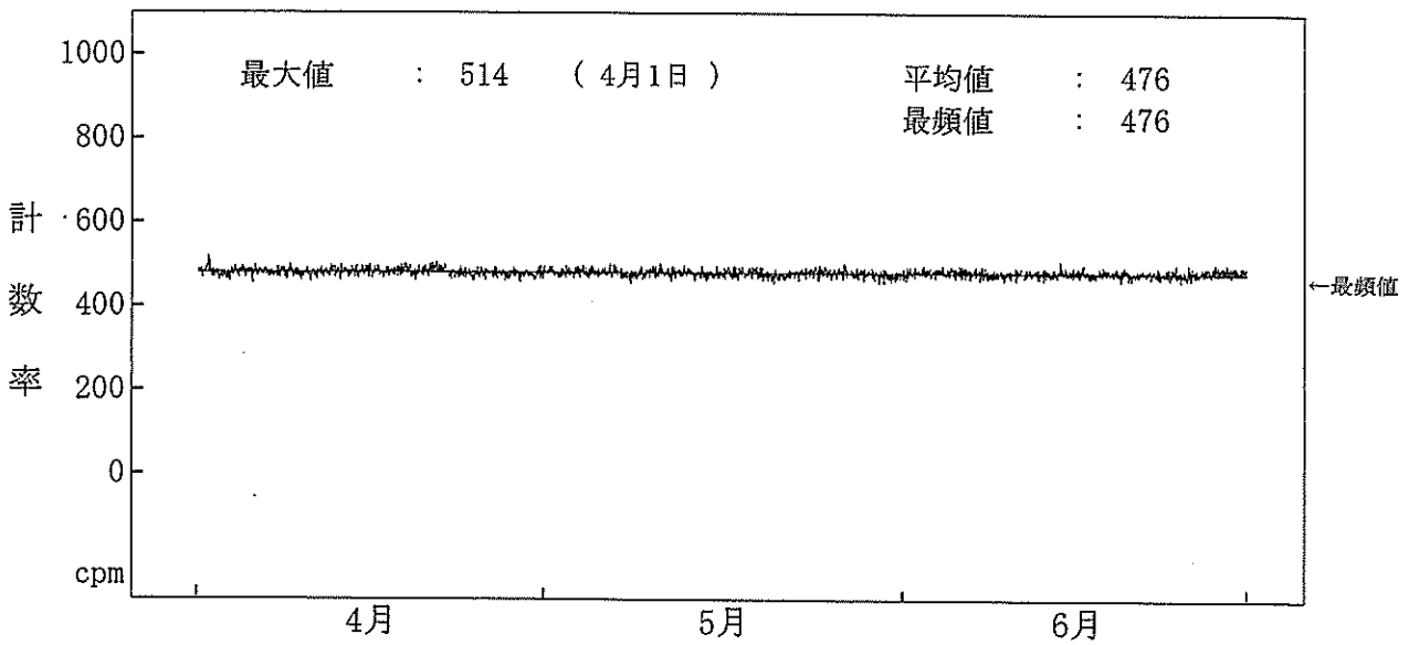
図-2-15 海水(放水)中の全ガンマ線計数率監視結果(3号機放水口モニター) (注) 4月22日、5月27日及び6月11日の欠測は、定期点検によるものである。
