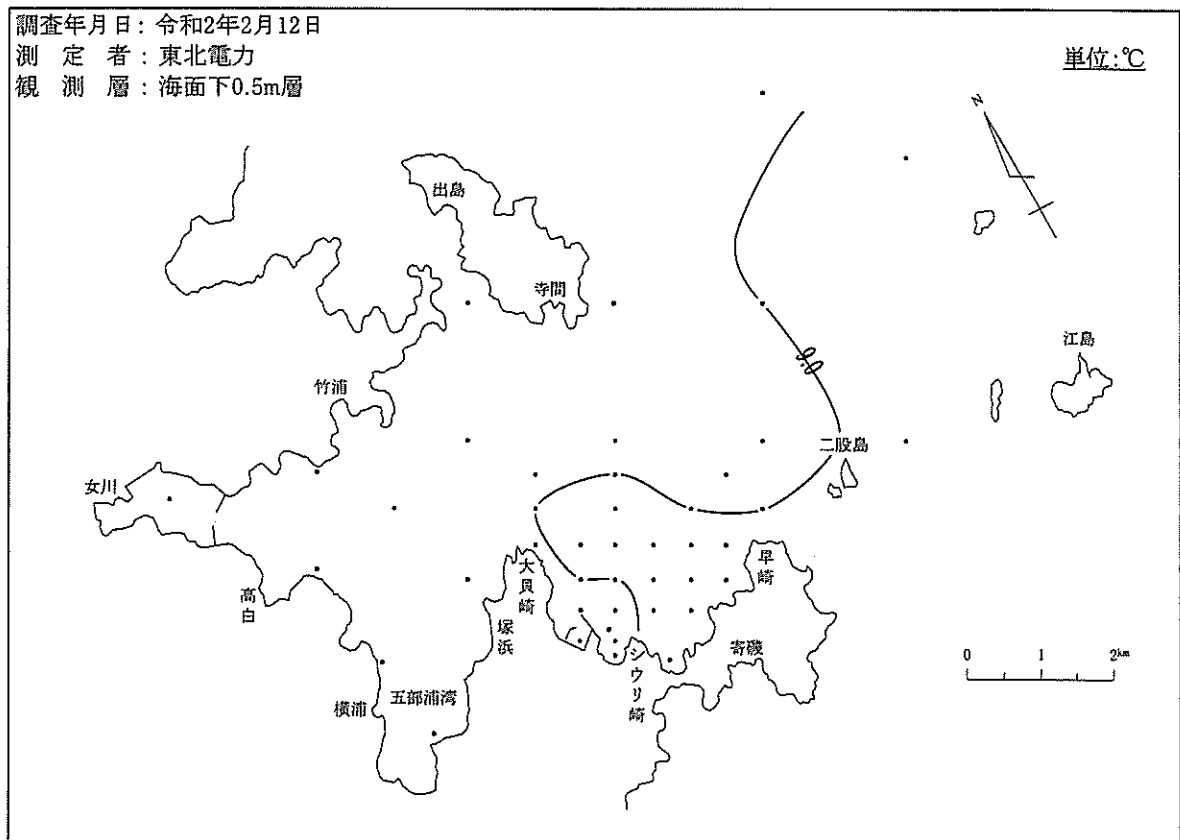
図-4-(2) 等温線
