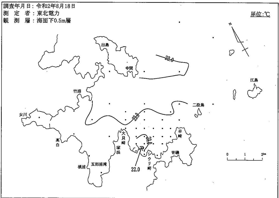
図-4-(2) 等温線
