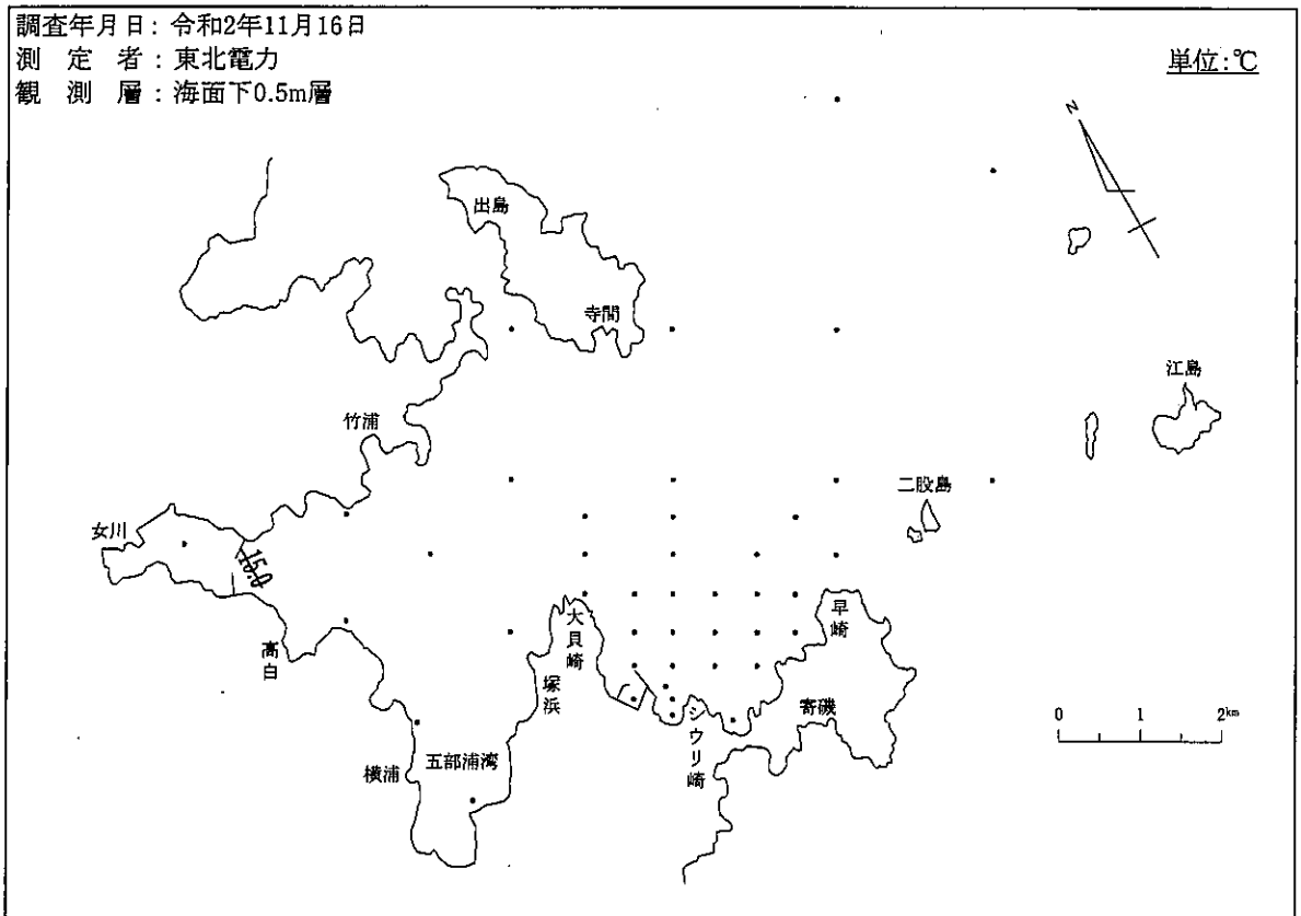
図-4-(2) 等温線
