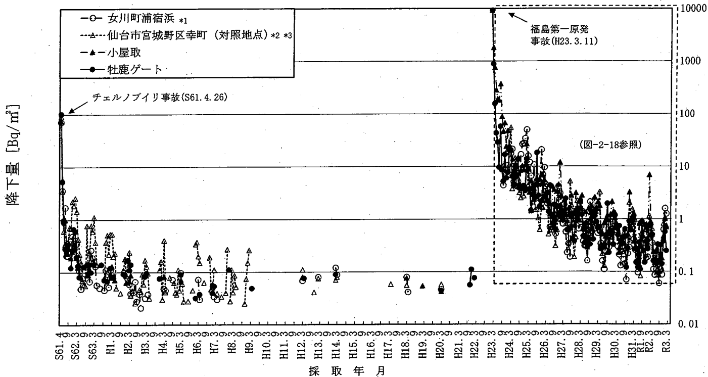
図-2-16 Cs-137の月間降下量の推移
