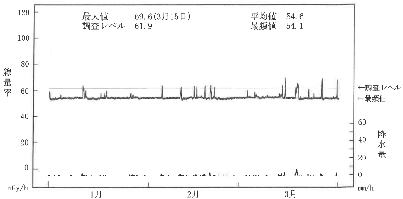
図-2-7 空間ガンマ線量率監視結果 (茨浜局)
