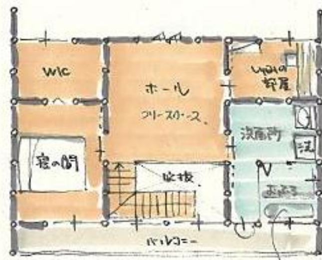
▲2階プラン
