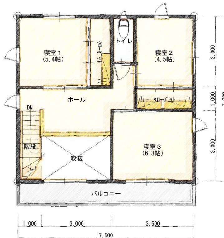
2階平面図
