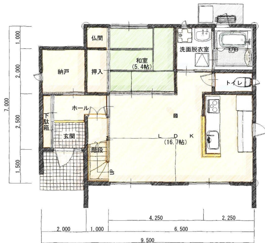
1階平面図
