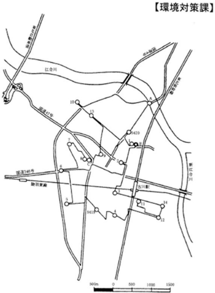
▼図3-4-3-2 古川地域水準測量観測路線
