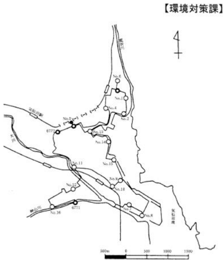
▼図3-4-3-3 気仙沼地域水準測量観測路線
