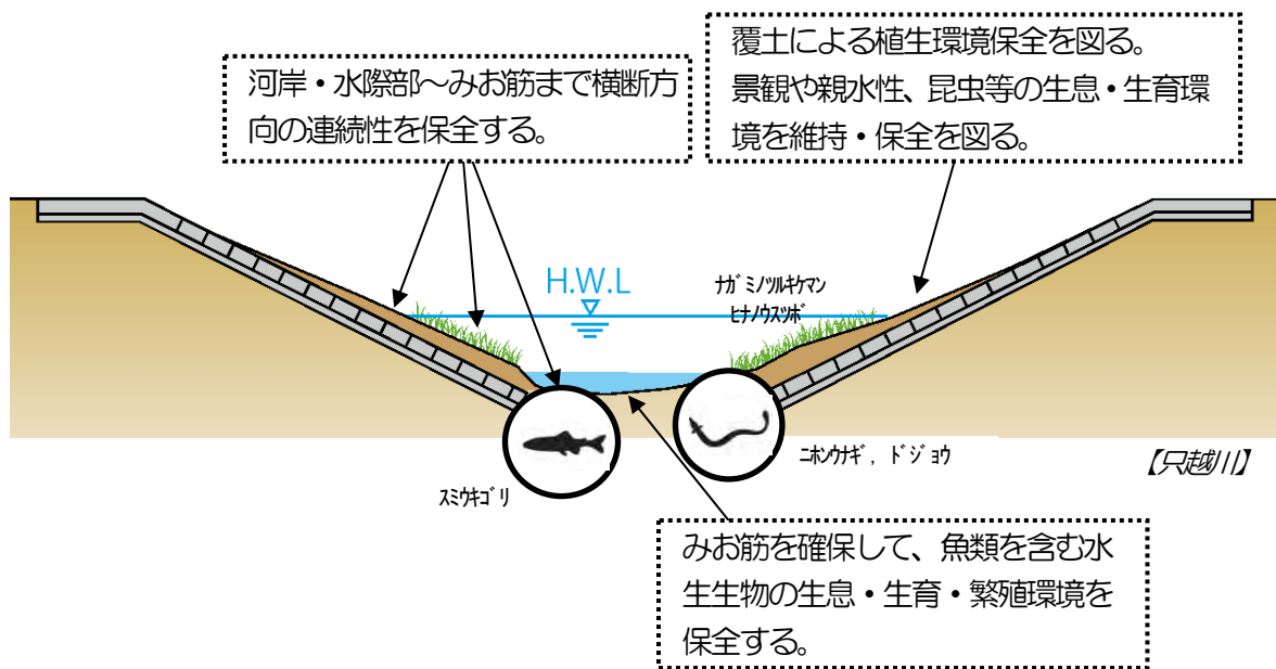
図 2-1 改修後の河川環境イメージ図
