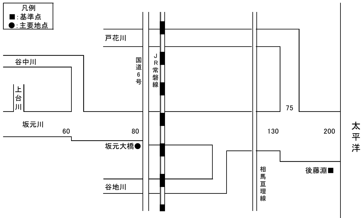
図 2-1 坂元川計画高水流量配分図
