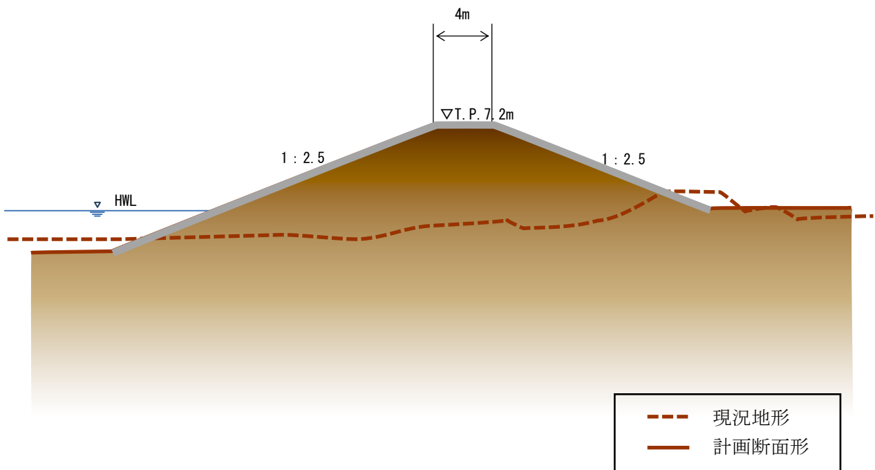
図 2-9 高潮、津波遡上に対応できる堤防整備イメージ
