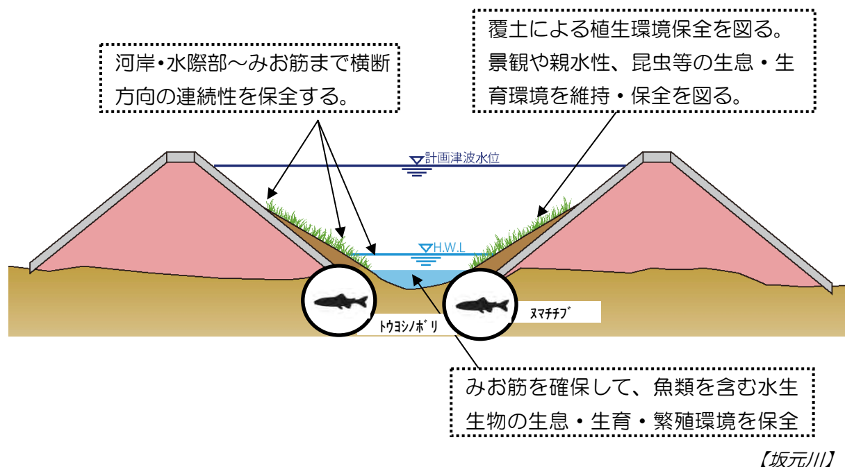
図 2-10 改修後の河川環境イメージ図
