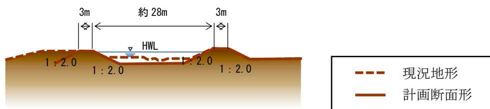
図 2-8 戸花川標準横断面図 (B 地点)
