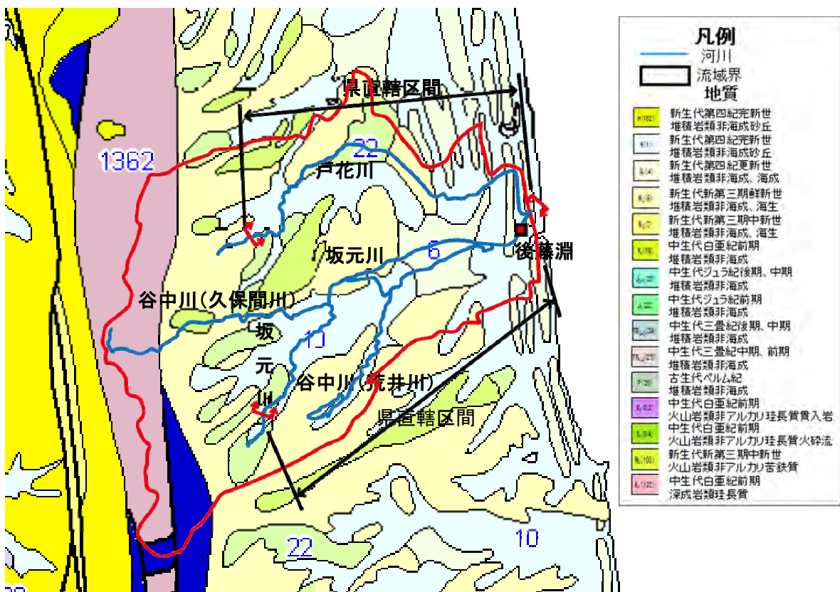
図 1-3 表層地質図
