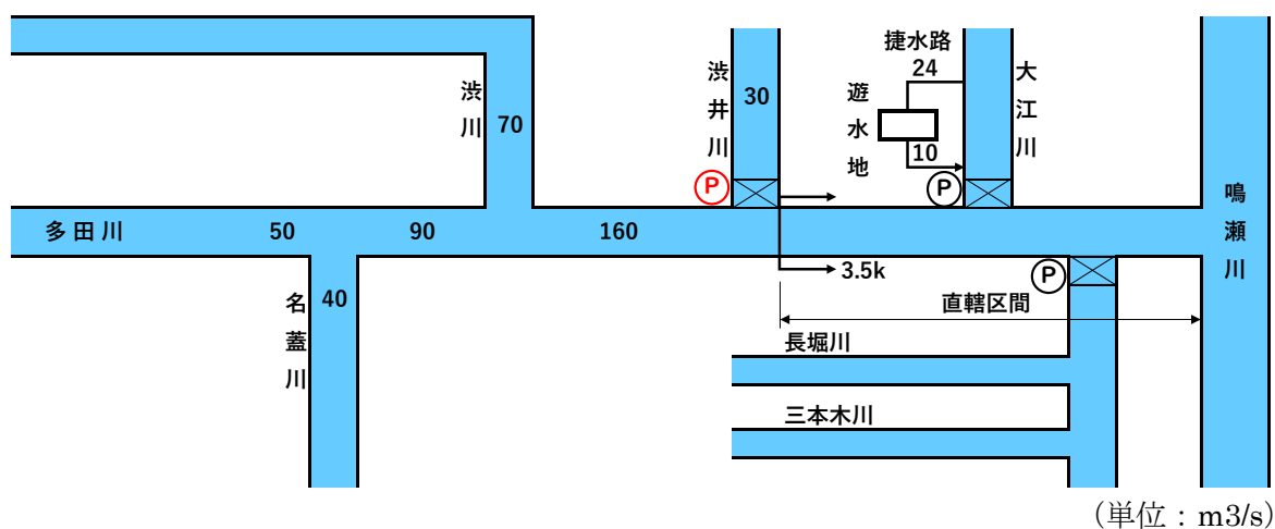
図 18 流量配分図
