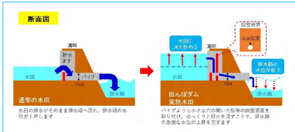
図 35 田んぼダム概要
