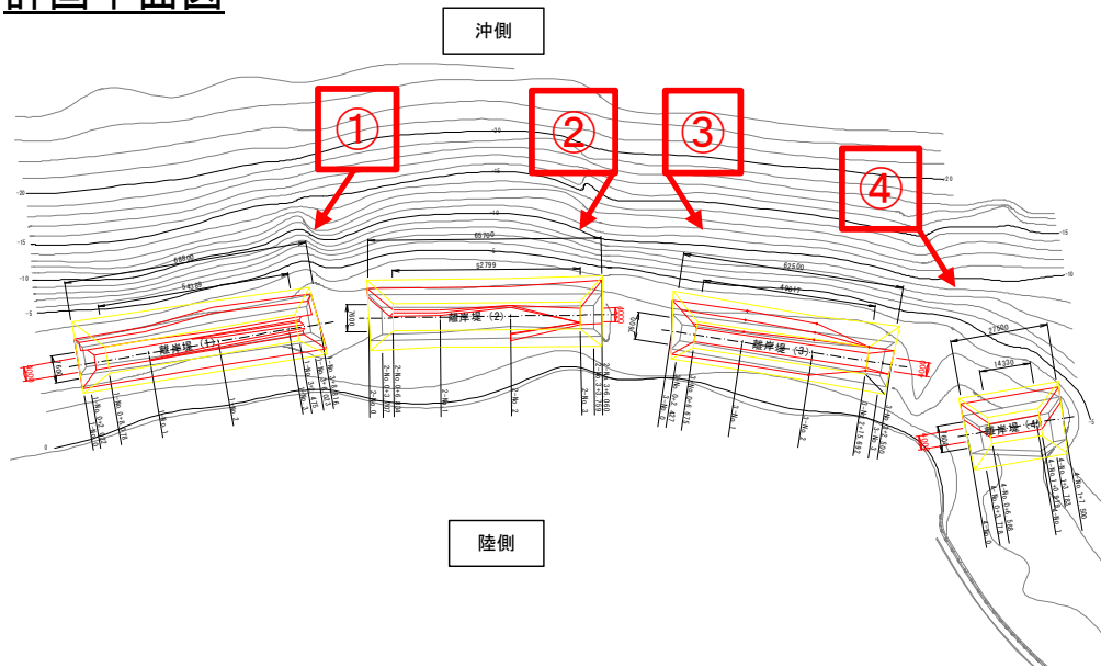
離岸堤(1)
