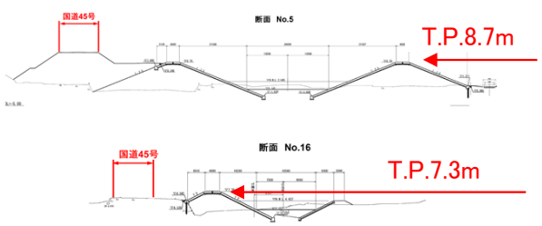
折立川 標準断面図
