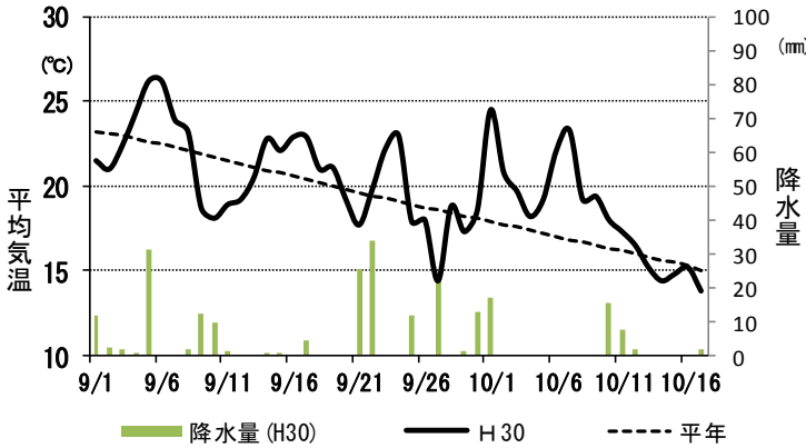
(1) 平均気温の推移（仙台アメダス）
