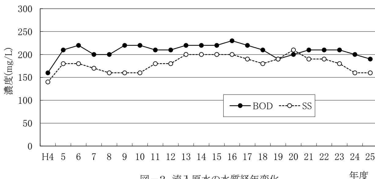
図一2 流入原水の水質経年変化
