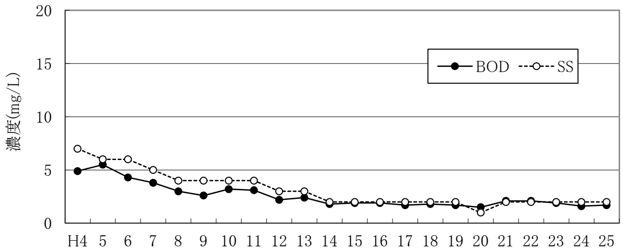
図-3 放流水の水質経年変化 年度
