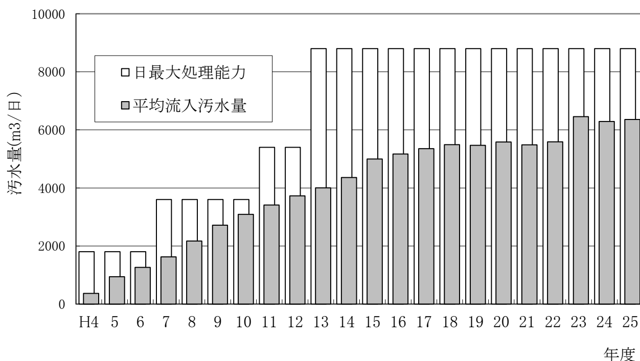
図一1 平均流入汚水量と日最大処理能力の経年変化
