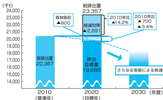
▲図3-1-1-1 温室効果ガス排出目標量と削減量
