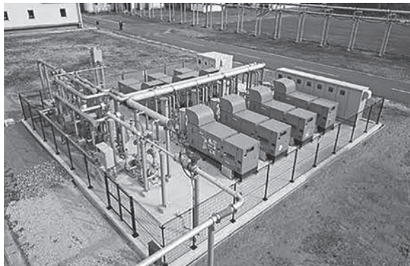
▲仙塩浄化センター消化ガス発電所
