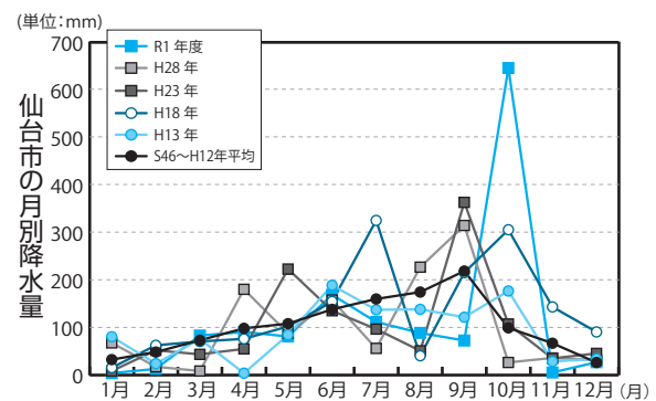
▲図 3-1-1-2 仙台市の月別降水量の推移 (出典：気象庁 HP)
