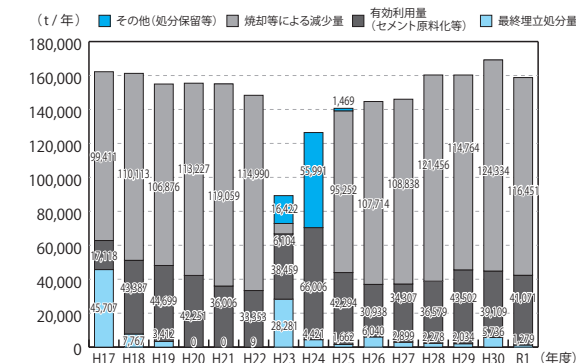
▲図 3-2-2-4 県内の下水汚泥処理の状況
