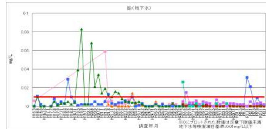
図 2-25 鉛（地下水）
