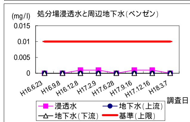
図 処分場内の浸透水採取設備及び場外の地下水観測井から採取した試料の経時変化(平成16年度以降)
