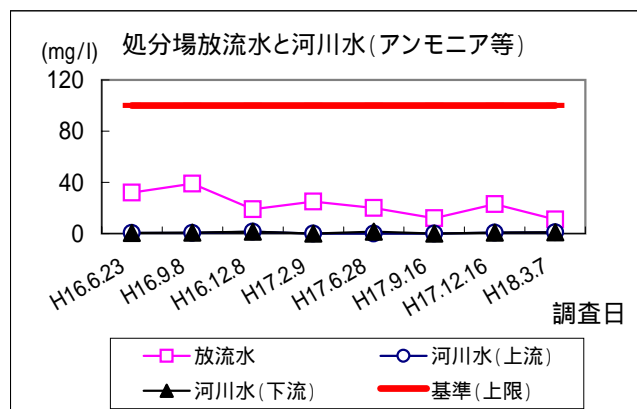
図 処分場の東側側溝末端及び流入する河川から採取した試料の経時変化(平成16年度以降)
