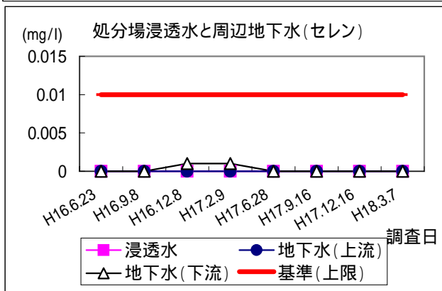
図 処分場内の浸透水採取設備及び場外の地下水観測井から採取した試料の経時変化(平成16年度以降)
