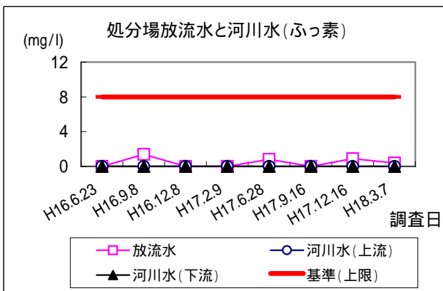
図 処分場の東側側溝末端及び流入する河川から採取した試料の経時変化(平成16年度以降)
