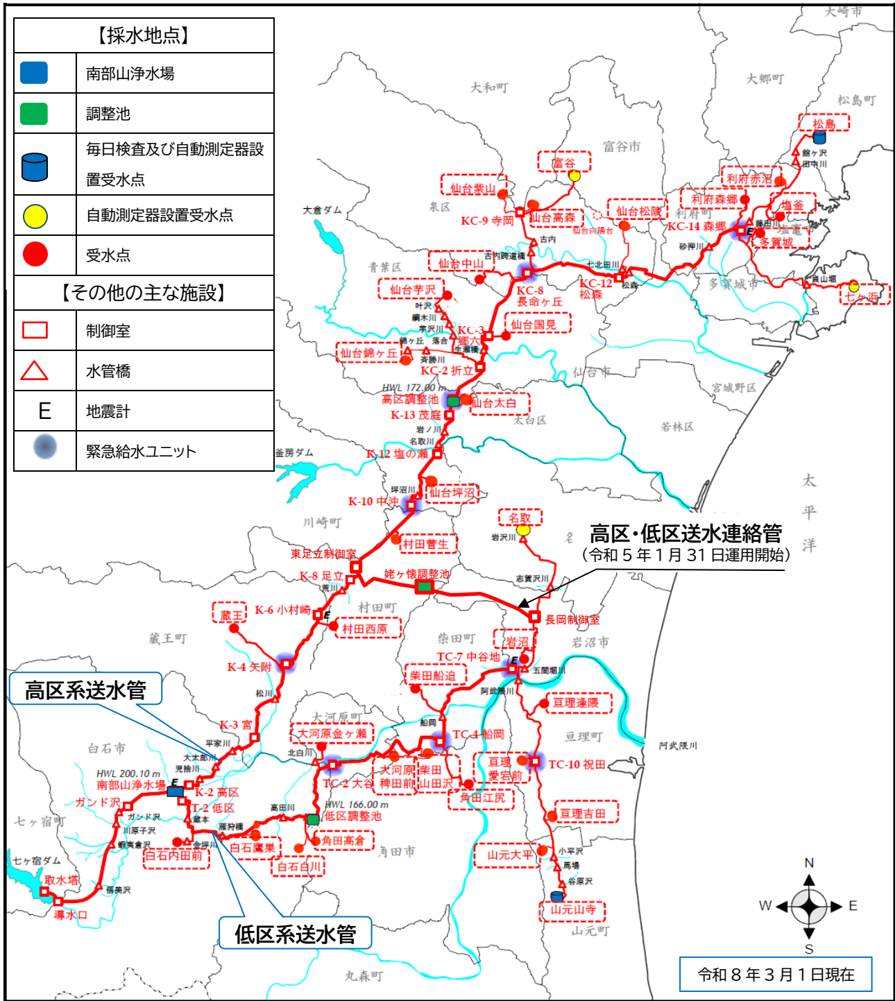
図1 管内概要図
