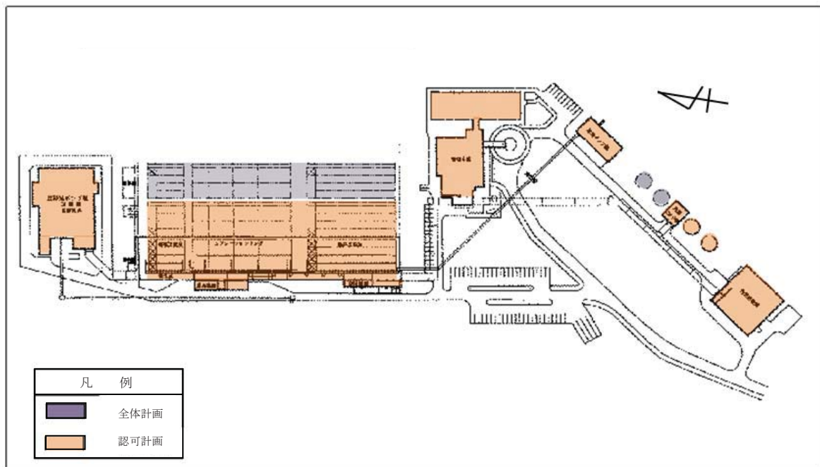
石巻浄化センター平面図
