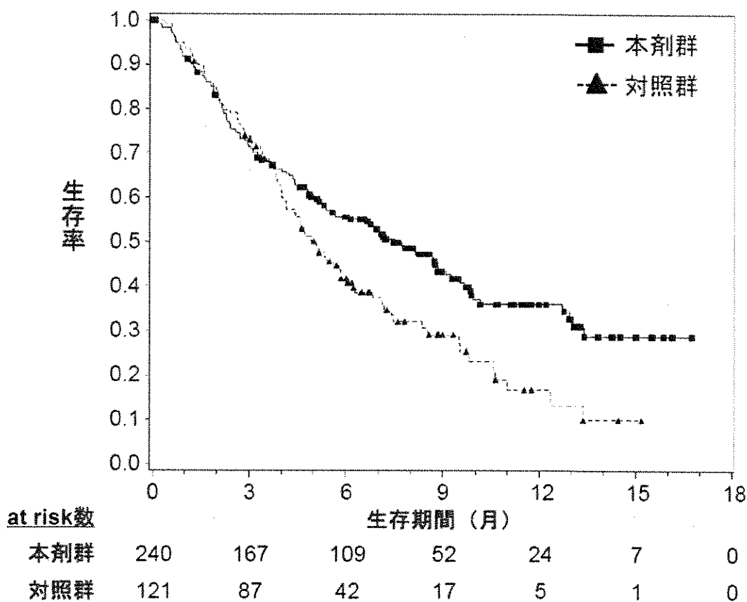
図1 OSのKaplan-Meier 曲線
