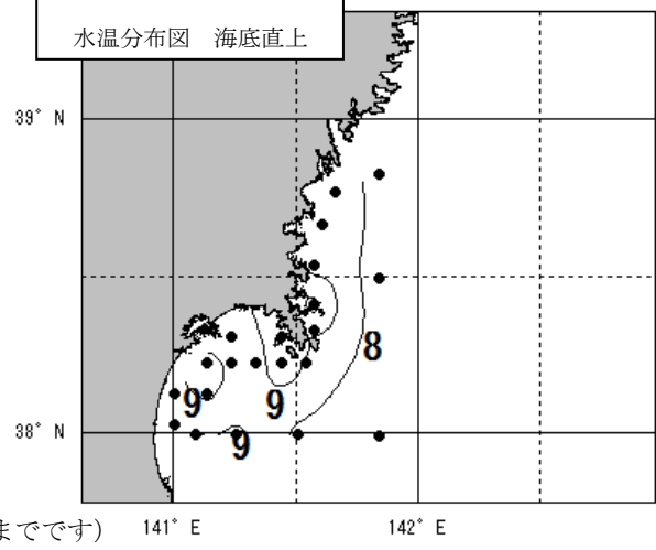
・海底直上水温(2018年4月3日～4月20日)
