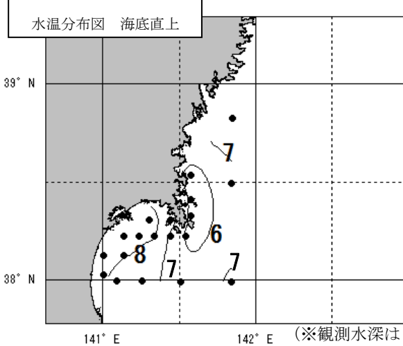
・海底直上水温(2019年4月17日～4月23日)
