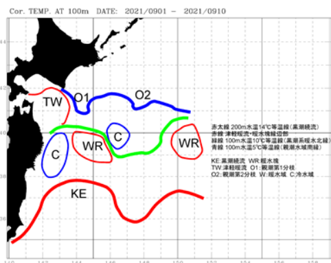
9月中旬予測水温分布
