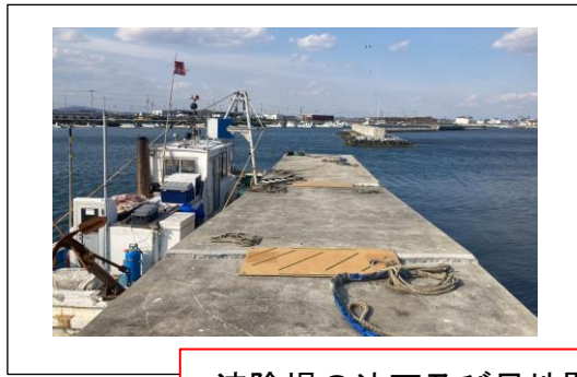
波除堤の沈下及び目地開き
