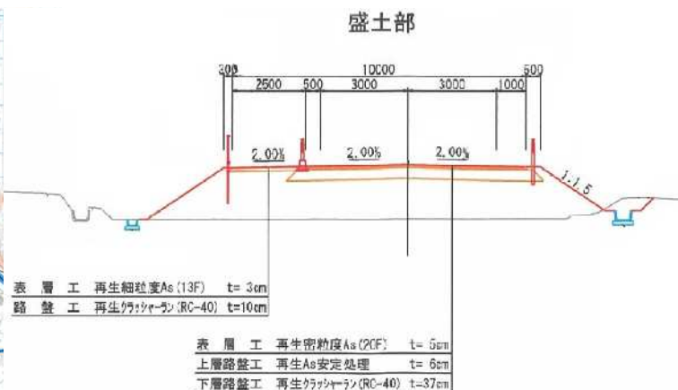
【標準横断面図】
