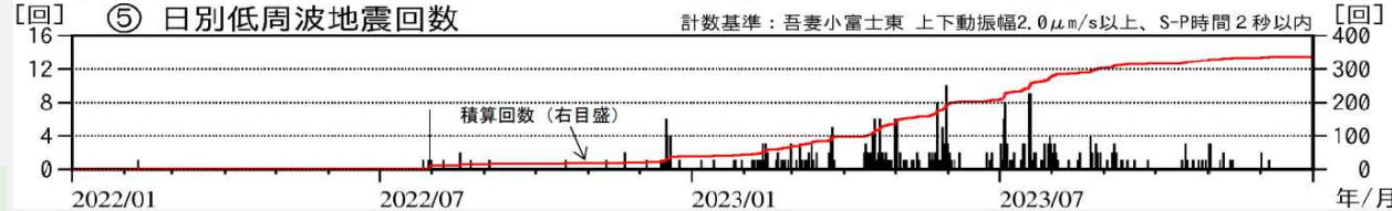
吾妻山の火山性地震（上），低周波地震（下）の日回数 （吾妻小富士東観測点）2022/1/1～2023/12/31
