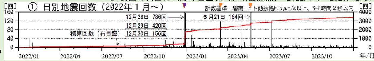
磐梯山の火山性地震の日回数（磐南観測点）2022/1/1～2023/12/31
