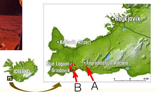
2023/12/18噴火 (B) (アイスランド気象庁)
