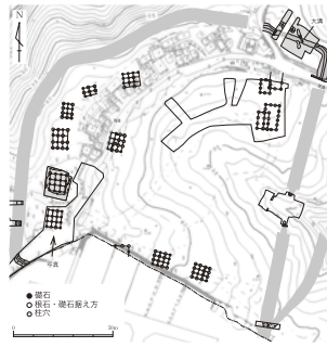
倉庫群配置図
