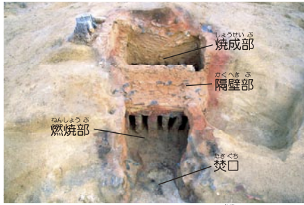
ロストル式の窯 全長4.6m
