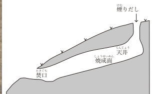
窯の模式図
