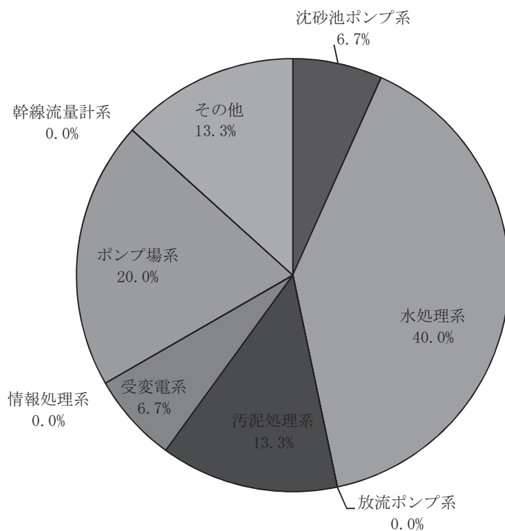
設備別故障発生割合
