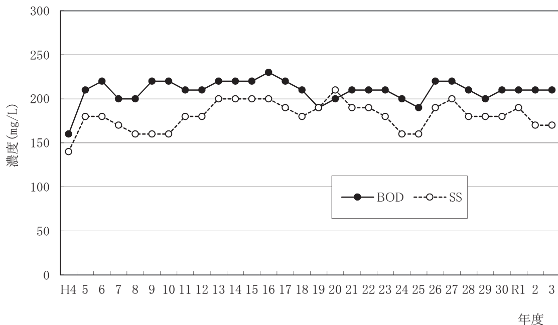
図一2 流入原水の水質経年変化
