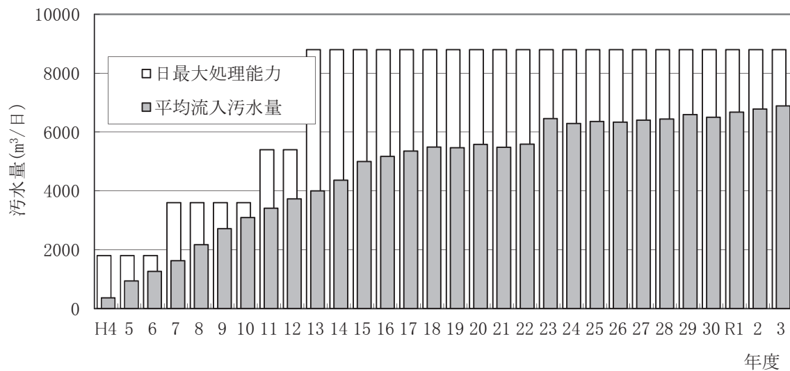
図一1 平均流入汚水量と日最大処理能力の経年変化
