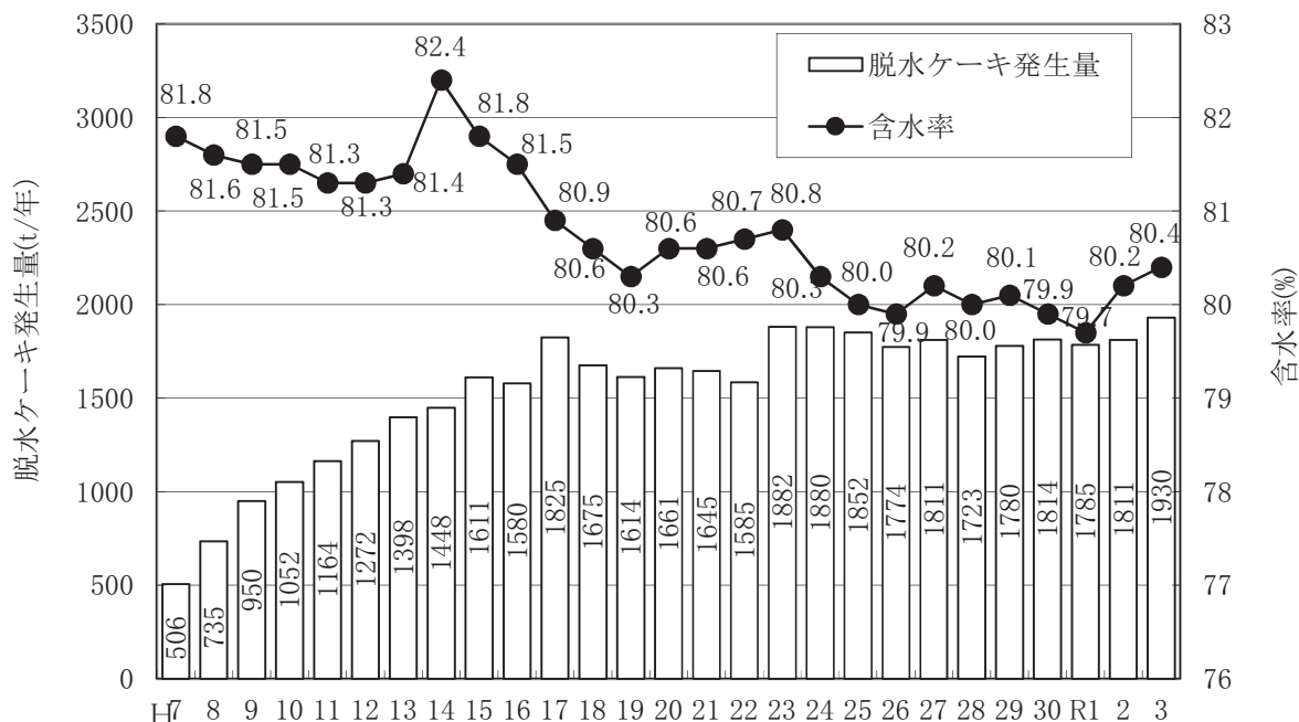
図-4 脱水ケーキ発生量及び含水率の経年変化 年度
