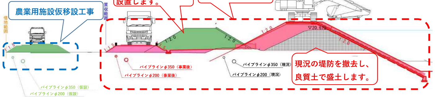
代表断面図
