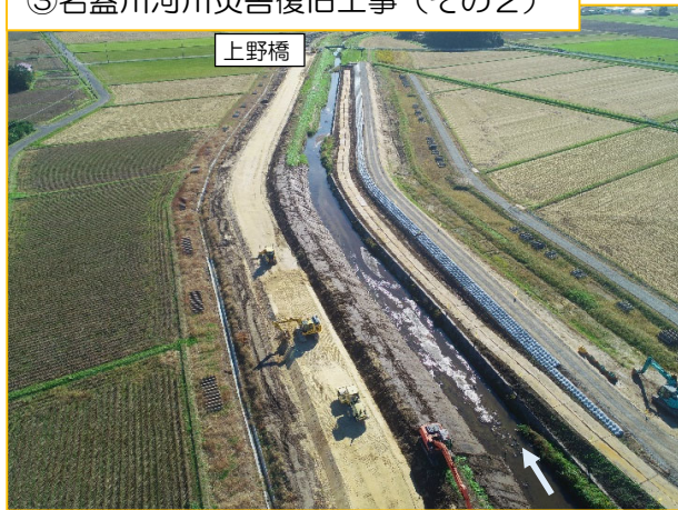
③名蓋川河川災害復旧工事（その2）
