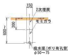
吸水渠断面
