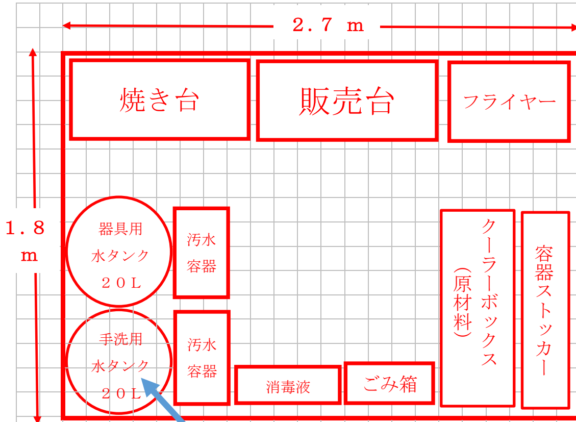
営業施設の平面図（一目盛 m）
