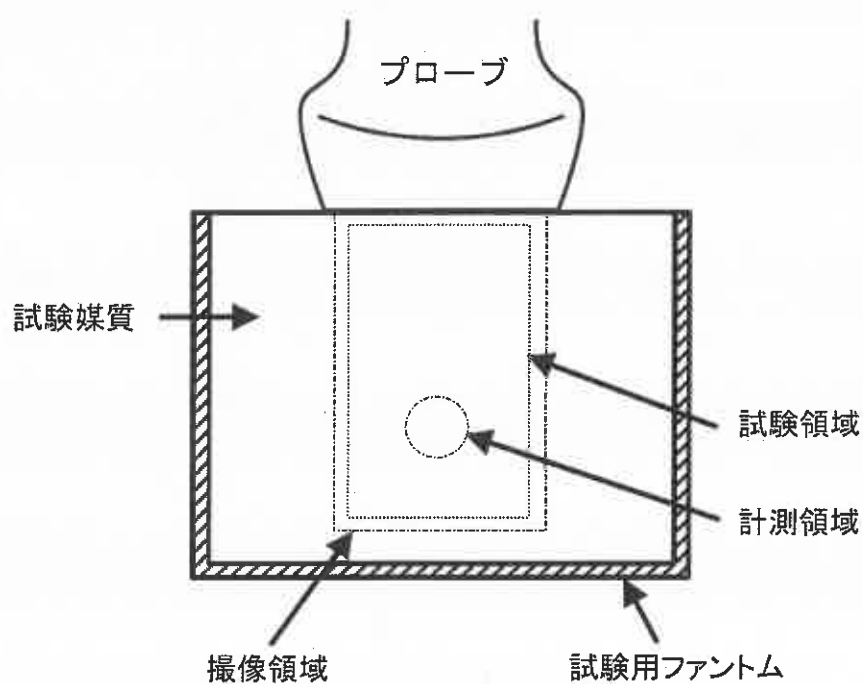
図 2 ー 超音波減衰係数計測の模式図(例) (計測領域を指定する機能がある場合)
