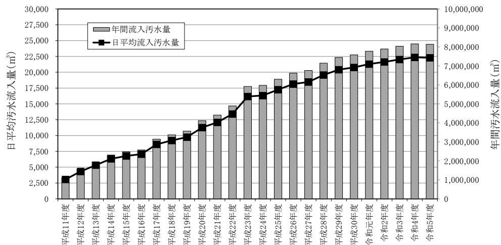
汚水流入量の経年変化(石巻浄化センター)
