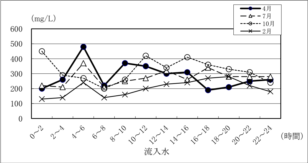
BOD 通日試験結果
