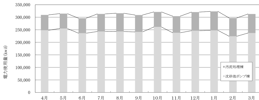
月別電力使用量(石巻浄化センター)
