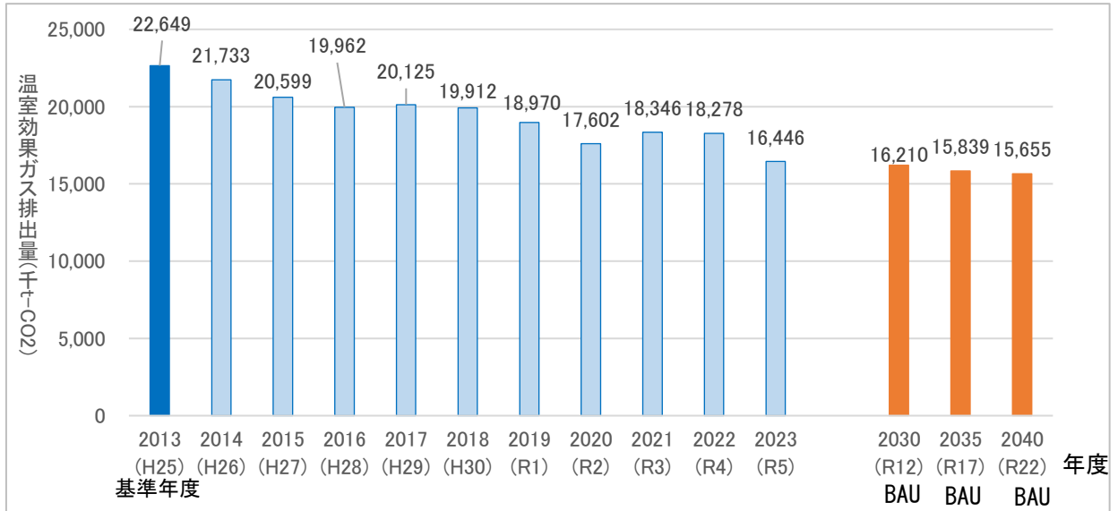
図 2-5 温室効果ガス排出量の将来推計
