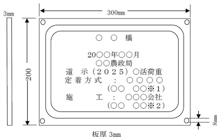
図 12-4-1 橋歴板の記載例
