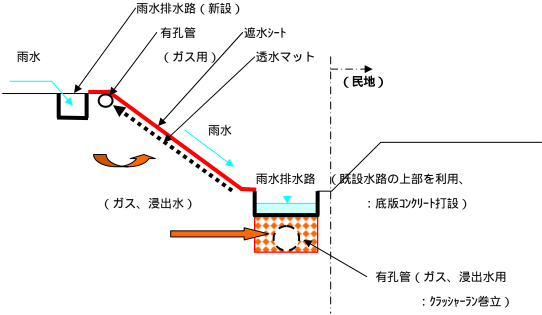
図 6-3-2 緊急対策工概念図 (横断面図)
